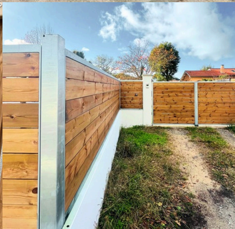
Modèle SABLE-cadre galvanisé à chaud + remplissage lames pin
