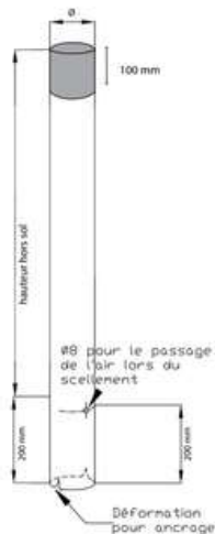
Option : bandes réfléchissantes
