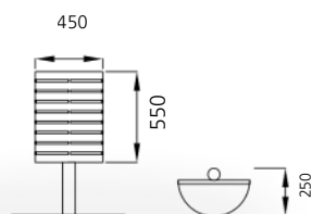
1/2 ZEPHIRIN SUR POTELET OU MURALE.
